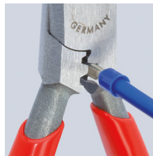
Опрессовка от 0,5 до 2,5 мм 2
